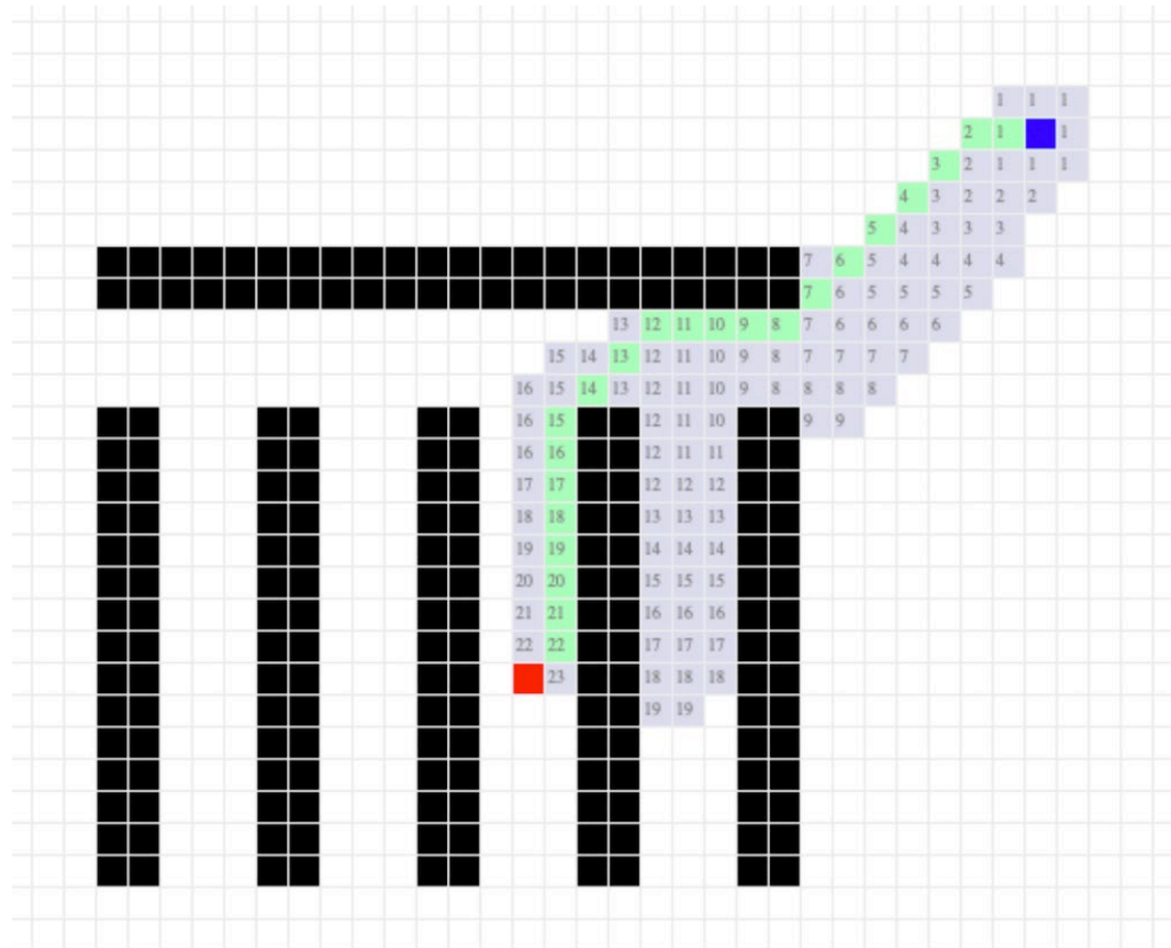
A-star
